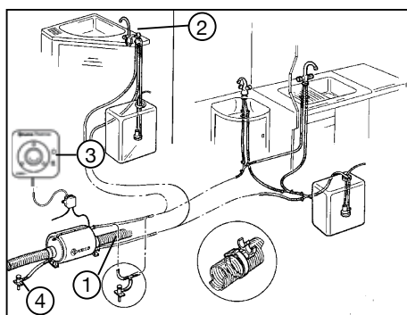
Schema dell'alimentazione di acqua calda
